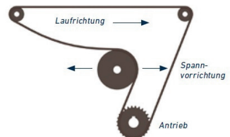
„S“-Antrieb
