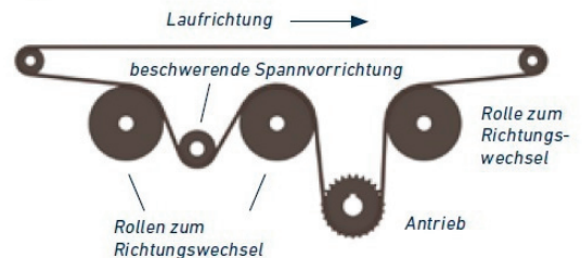
Omega-Antrieb
